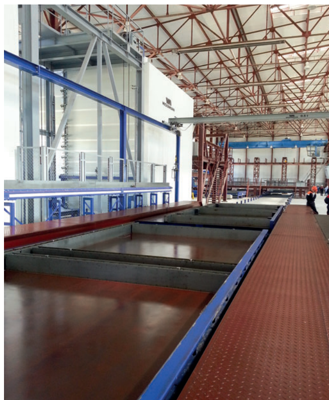
A nova instalação de circulação para elementos de concreto pré-moldado, que a Weckenmann construiu no Cazaquistão, é generosamente dimensionada.
